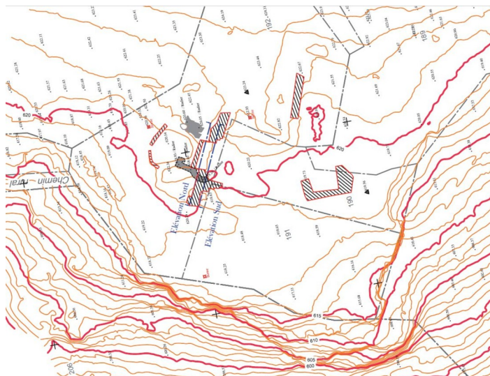
Plan géomètre
